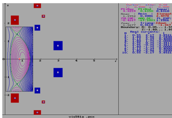
Рис. 2. Равновесие в токамаке STF, рассчитанное по старой версии кода
