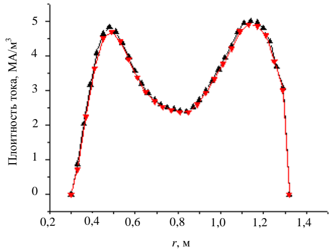
Рис. 1. Сравнение плотности тока, вычисленной с помощью кода ТОКАМЕQ (▲) и кода УКАЕА (▼) института (Великобритания)
