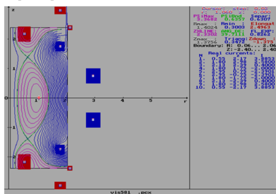
Рис. 3. То же равновесие, что на рис. 2, рассчитанное по новой версии кода
